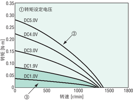
转速—转矩特性例
