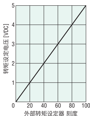
外部转矩设定器刻度—转矩设定电压特性（代表值）
