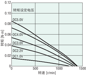
2TK3GN-CW2E、2TK3A-CW2E (230V 50Hz)
