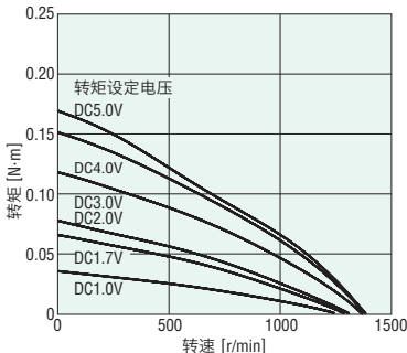
3TK6GN-CW2E、3TK6A-CW2E (230V 50Hz)
