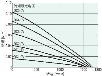
2TK3GN-CW2E、2TK3A-CW2E (220V 60Hz)
