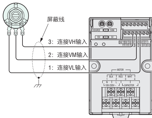
外部转矩设定器 PAVR-20KZ（另售）
