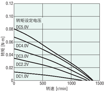
2TK3GN-CW2E、2TK3A-CW2E (220V 50Hz)
