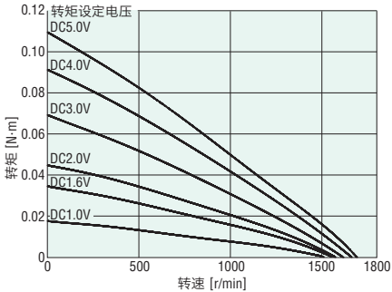
2TK3GN-CW2E、2TK3A-CW2E (230V 60Hz)
